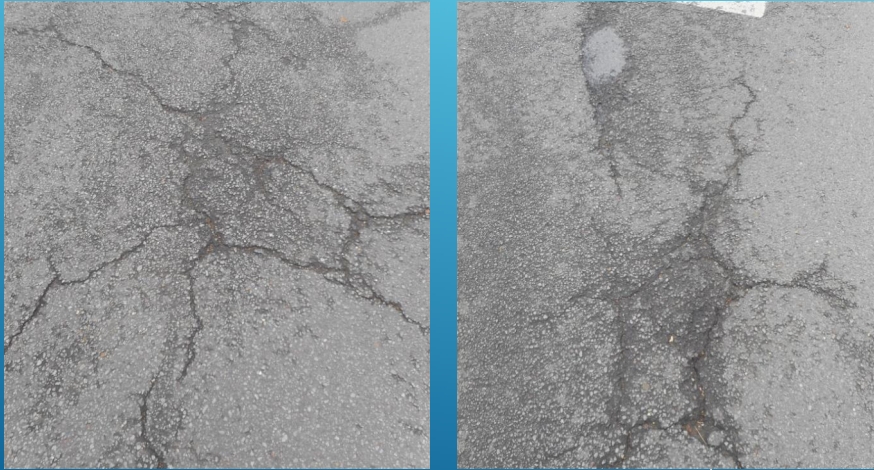
Netzrisse, Ausbrüche
