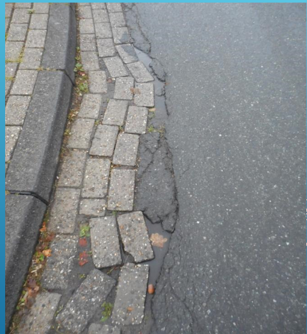
Abgängige Rinnen
